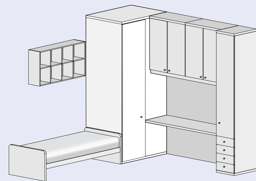
ZONA RIPOSO + KUBO + PONTE SLEEPING AREA+KUBO+BRIDGE
